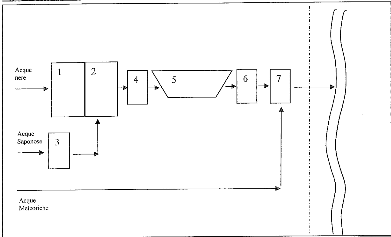
Fig. 2 Schema tipo scarico fuori fognatura
